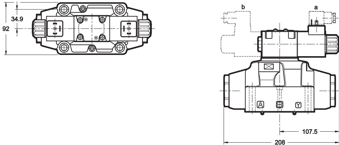
DSP7-TA DSP7-SA* положение электромагнита в конфигурации ТВ/*SB
