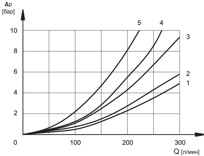
ПАДЕНИЕ ДАВЛЕНИЯ ПРИ ИНИЦИИРОВАННОМ КЛАПАНЕ
